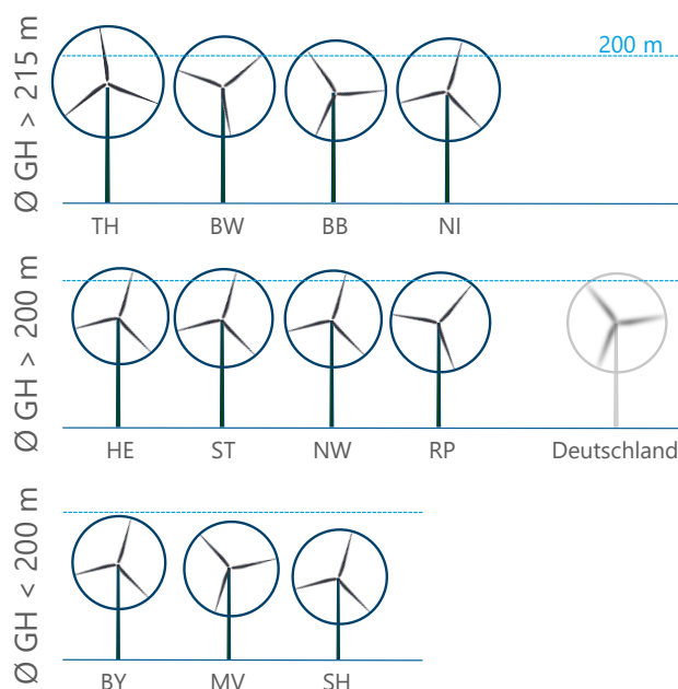
Anlagenkonfiguration des Zubaus in den Bundesländern
